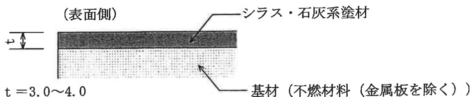
図1 断面図
